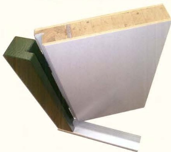
Querschnitt durch eine Ganzblatt-Tür mit umlaufendem Stahlkern
